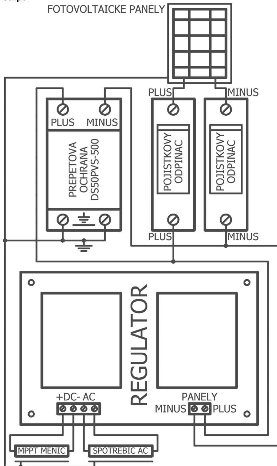
Doporučené schéma zapojení pro 1. a 2. režim činnosti
