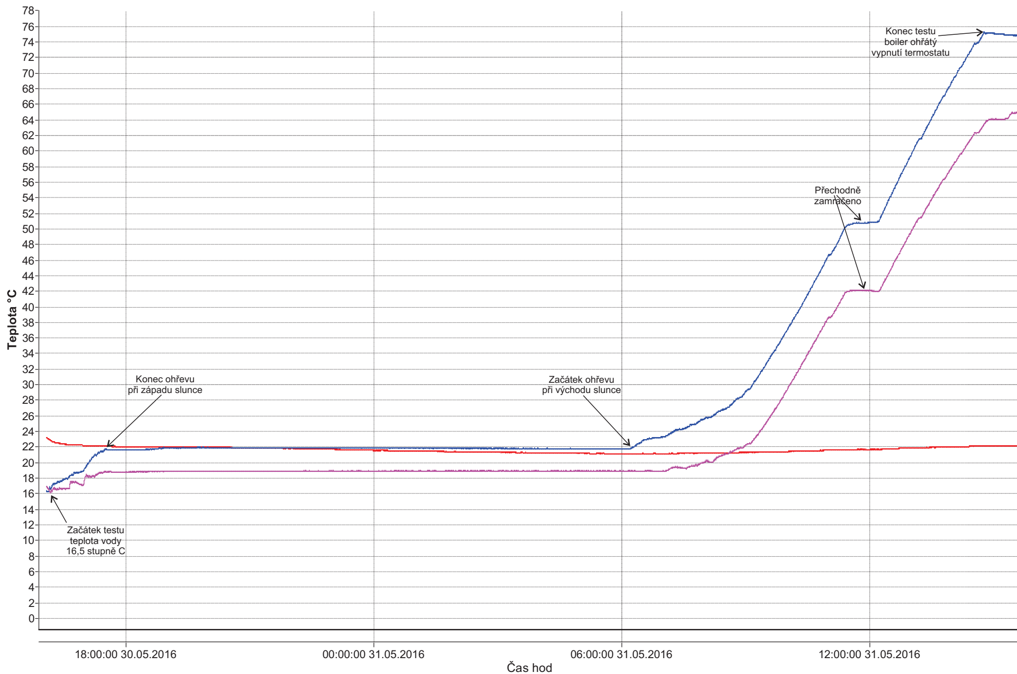
Graf teploty vody v boilerech při napájení z MPPS (modrá křivka) a MPPT regulátoru (fialová křivka). Regulátory byly napájeny stejným počtem panelů umístěných na jedné střeše ve stejném čase.
