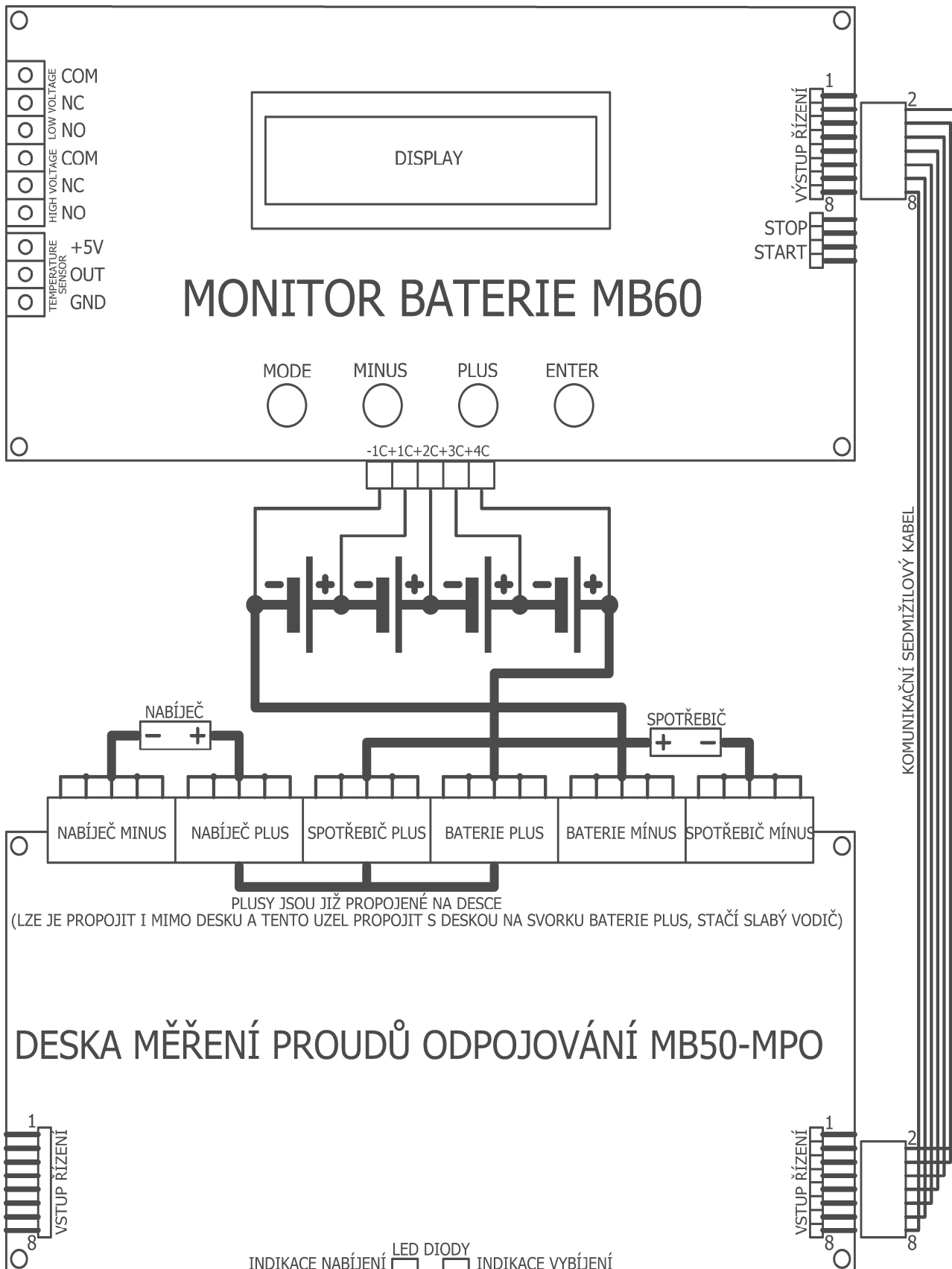
Schéma spojení desek
